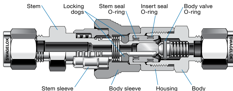
Single-End Shutoff (SESO)
